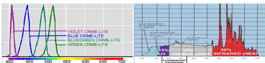
مقایسه بازه طول موج تولیدی لامپ های Xenon (تصویر سمت راست) با لامپ های LED (تصویر سمت چپ)
